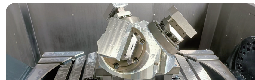
4/5軸構造が複雑な部品加工に対応可能
