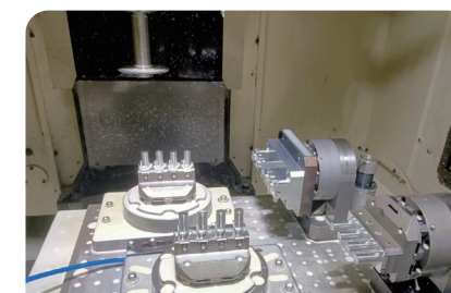
自己研磨を用いたゼロクランプシステム
